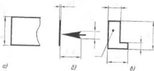
Рис. 29. Нанесение линейных размеров
