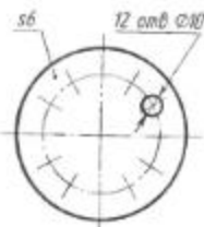
Рис. 205. Изображение одинаковых, равномерно расположенных элементов
