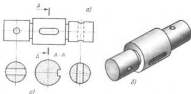
Рис. 163. Валник
