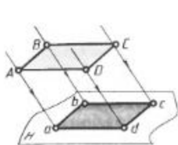
Рис. 41. Косоугольное проецирование
