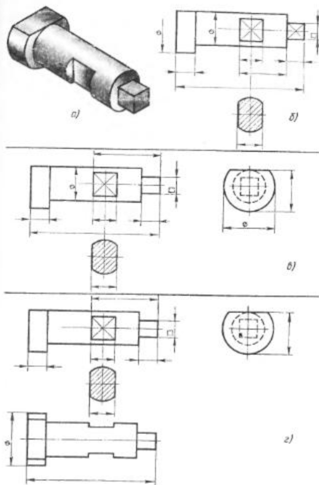
Рис. 203. Определение рациональности выполнения чертежа
