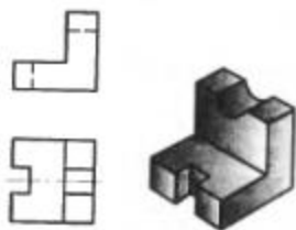
Рис. 48. Неопределенность формы предмета на изображении
