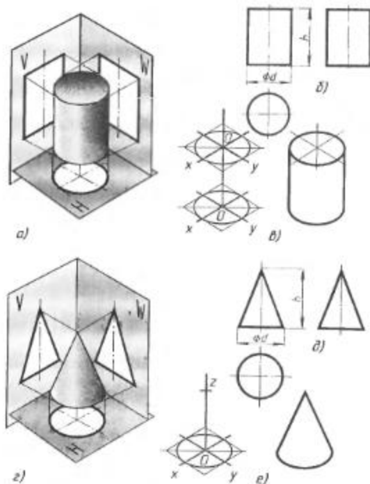
Рис. 80. Цилиндр и конус:
