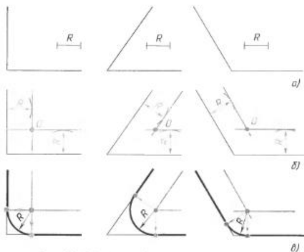
Рис. 132. Общий способ построения сопряжений двух пересекающихся прямых
