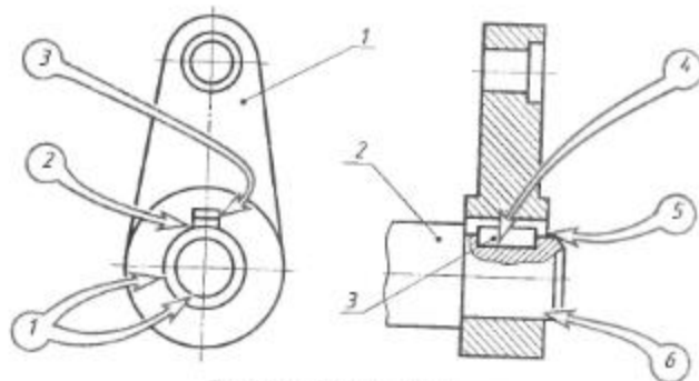
Рис. 226. Чертеж для чтения
