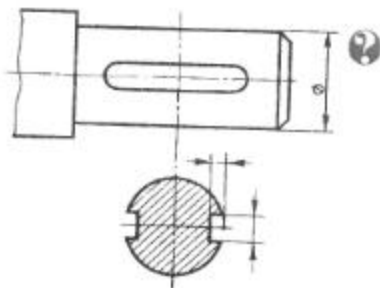
Рис. 175. Пример нанесения размеров на сечении
