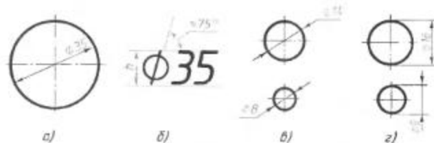
Рис. 30. Нанесение размера окружностей
