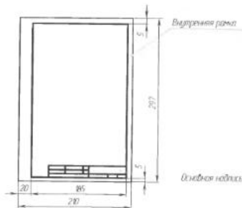
Рис. 18. Оформление листа формата А4
