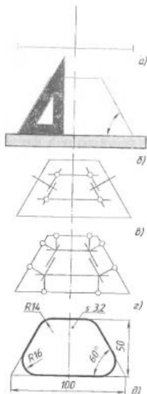
Рис. 135. Последовательность построения чертежа шаблона
