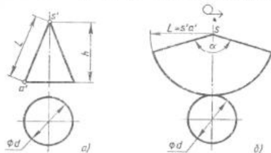
Рис. 141. Построение чертежа развертки поверхностей конуса: a — диаметр; b — развертка поверхностей
