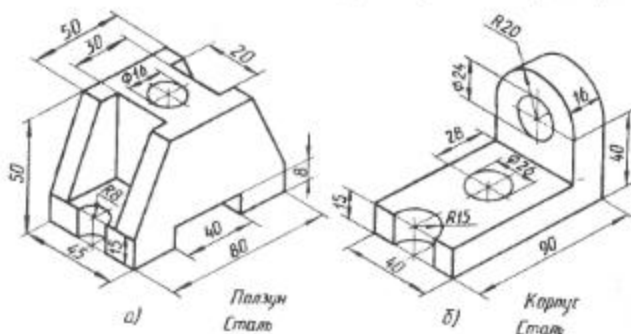
Рис. 200. Задания для графической работы № 13
