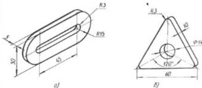
Рис. 138. Задания к графической работе № 6
