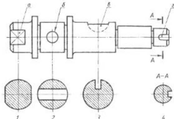
Рис. 168. Изображение, полностью выявляющее форму предмета
