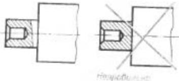
Рис. 190. Правильное и ошибочное выполнение местного разреза
