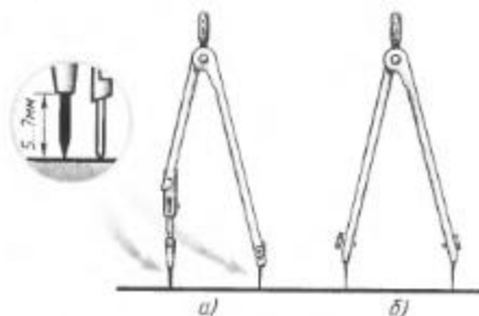
Рис. 11. Циркуль чертежный: а — круговой; б — разметочный
