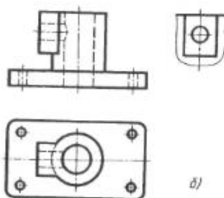
Рис. 54. Местные виды, разложенные в проекционный способ
