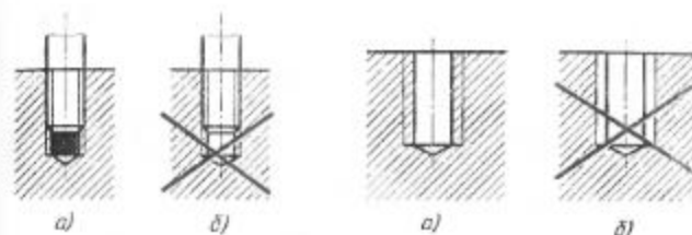
Рис. 220. Изображение шпильки, ввинченной в отверстие с резьбой: а — правильно; б — неправильно
