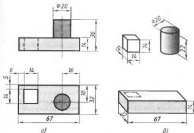
Рис. 116. Нанесение размеров
