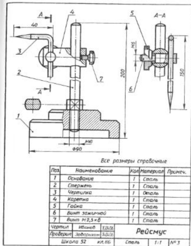
Рис. 238. Чертеж для чтения
