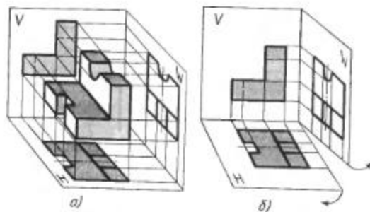
Рис. 49. Проецирование на три плоскости проекций
