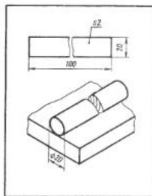
Рис. 156. Задание к графической работе № 10
