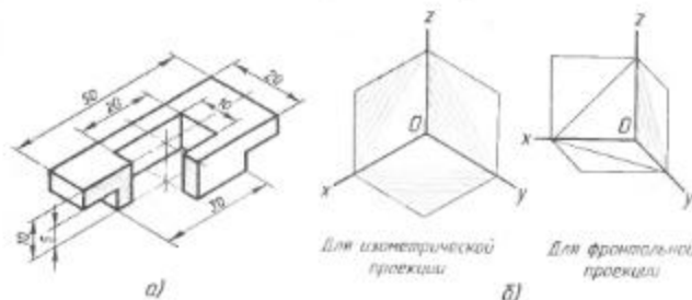
Рис. 199. Разрезы в аксонометрических проекциях
