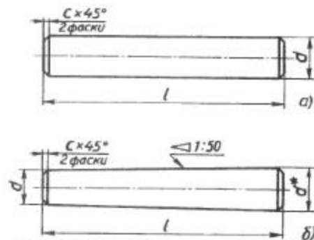
Рис. 227. Чертежи штифтов
