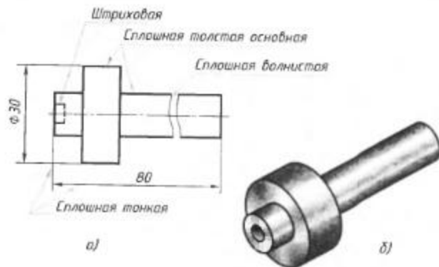
Рис. 21. Линии чертежа
