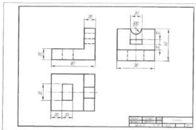
Рис. 6. Эскиз детали
