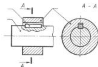
Рис. 224. Чертежи деталей шпоночного соединения
