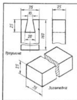
Рис. 157. Задание к графической работе № 10
