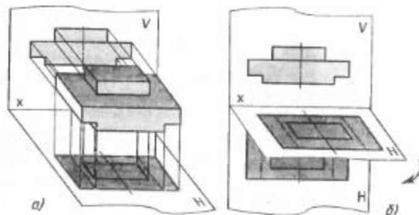
Рис. 46. Проецирование на две плоскости проекций
