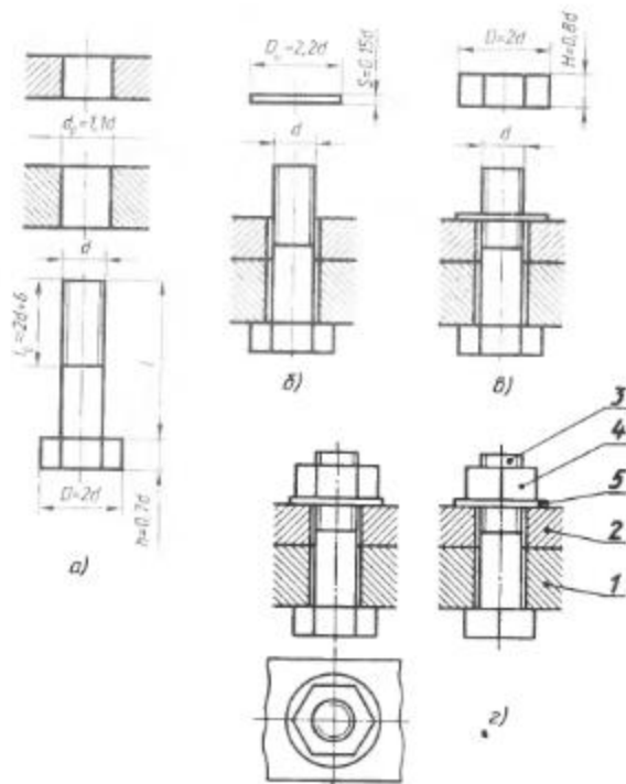
Рис. 217. Упрощенное изображение болтового соединения
