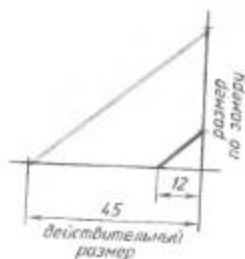
Рис. 258. Угловой (пропорциональный) масштаб
