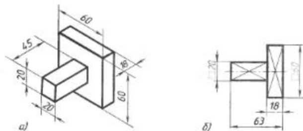
Рис. 77. Изображение детали в одном виде
