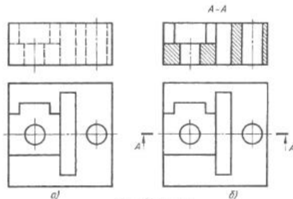
Рис. 166. Корпус
