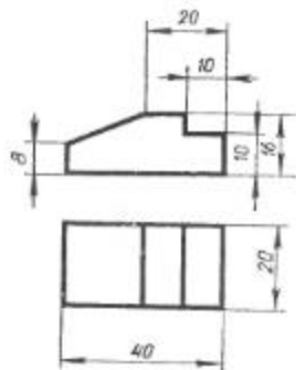
Рис. 62. Чертеж детали
