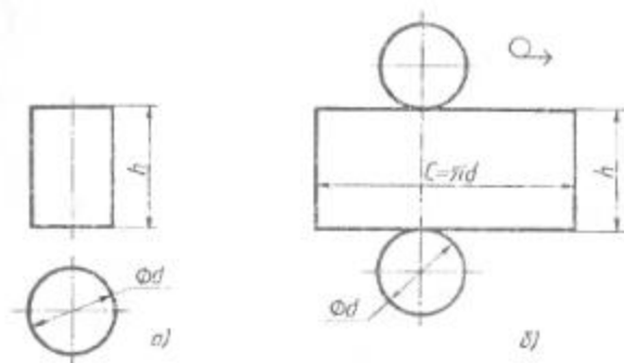
Рис. 140. Построение чертежа развертки поверхностей цилиндра: a — диаметр; b — развертка поверхностей
