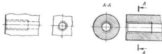
Рис. 212. Изображение резьбы в отверстии (без разреза)
