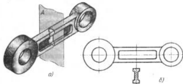
Рис. 169. Сечение: а — получение; б — изображение
