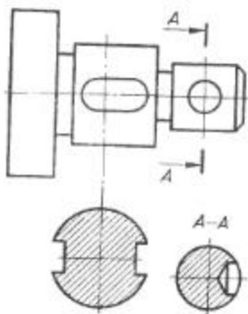
Рис. 170. Вынесенные сечения
