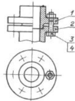
Рис. 243. Условное изображение повторяющихся элементов
