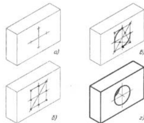
Рис. 68. Построение изометрической проекции детали с цилиндрическим отверстием
