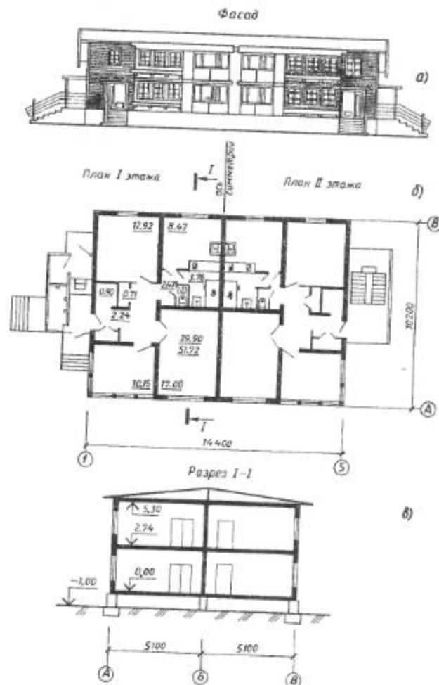
Рис. 260. Типовой проект здания
