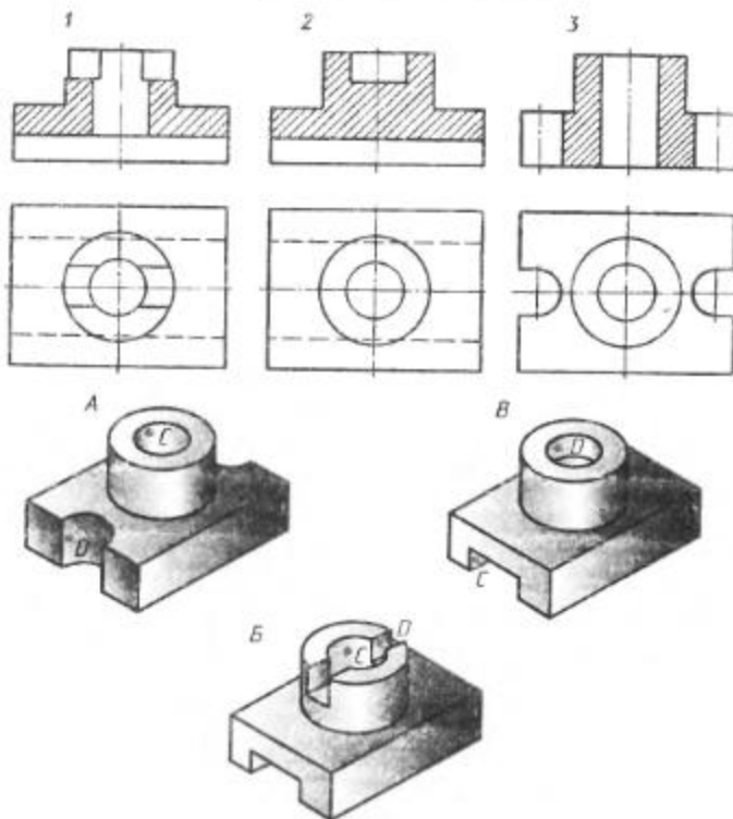
Рис. 180. Задание для упражнений
