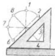
Рис. 125. Деление окружности на восемь равных частей
