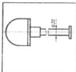
Рис. 159. Задание к графической работе № 10
