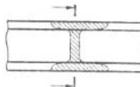
Рис. 172. Обозначение наложенного несимметричного сечения
