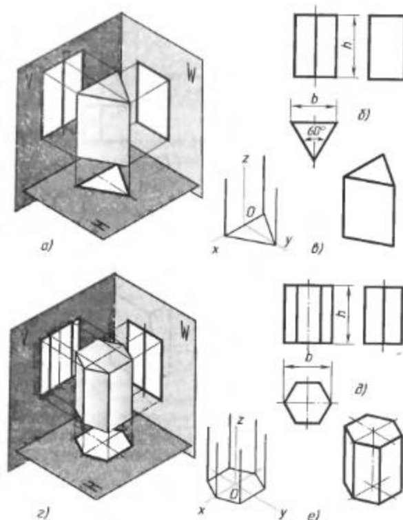
Рис. 78. Призмы:
