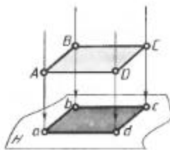
Рис. 42. Прямоугольное проецирование
