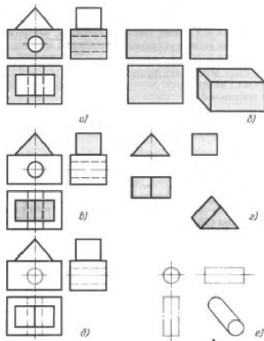
Рис. 101. Анализ формы детали
