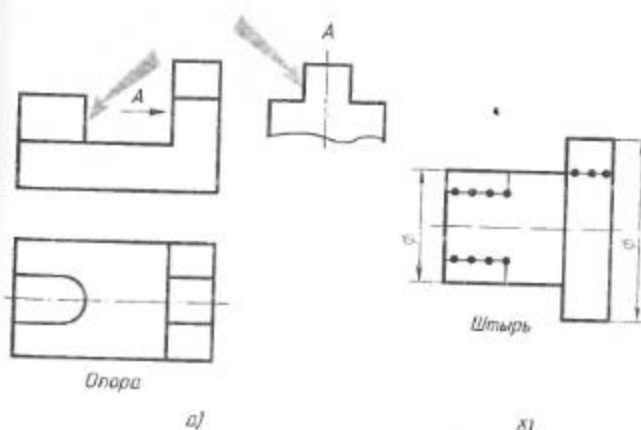
Рис. 149. Задания к графической работе № 8
