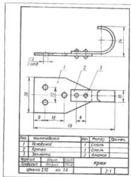
Рис. 5. Сборочный чертеж
