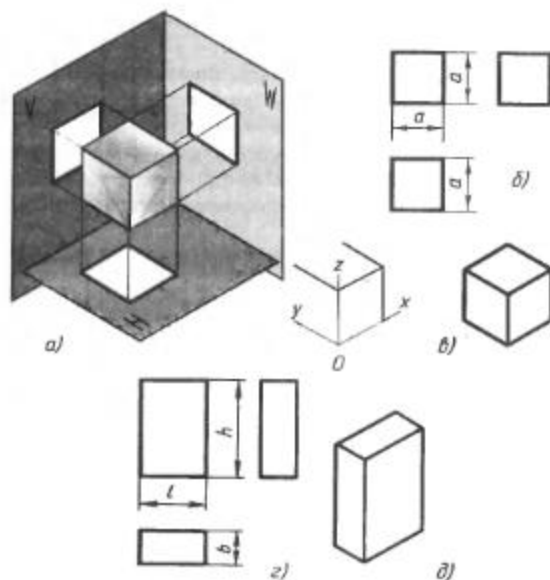
Рис. 76. Куб и прямоугольный параллелепипед: а — проецирование; б, в — чертежи в системе прямоугольных проекций; в, д — изометрические проекции *
