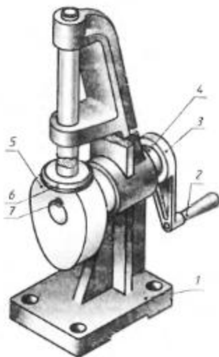
Рис. 231. Кулачковый механизм
