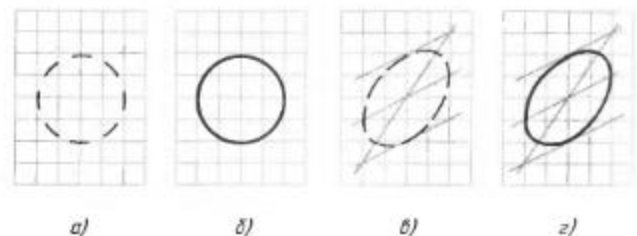
Рис. 70. Построения, облегчающие выполнение технических рисунков
