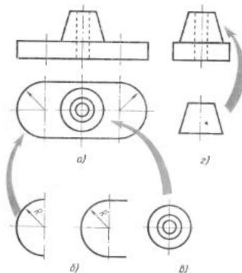
Рис. 123. Анализ графического состава изображений
