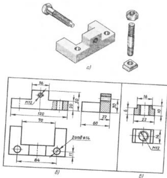
Рис. 251. Детали упора: а — наглядное изображение; б — чертеж детали «виноус»; в — чертеж детали «сухарь»
