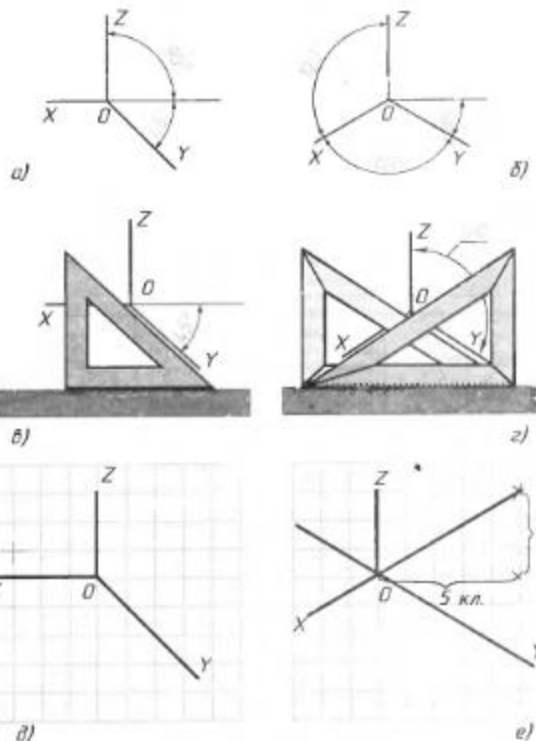
Рис. 61. Изображение осей аксонометрических проекций: а, б — положение осей; а, е — приемы построения осей; д, е — построение осей при выполнении технических рисунков
