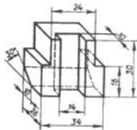
Рис. 102. Изядающее изображение опоры
