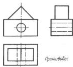
Рис. 100. Проекция детали
