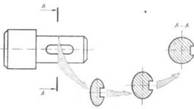
Рис. 173. Совмещение сечения с плоскостью чертежа
