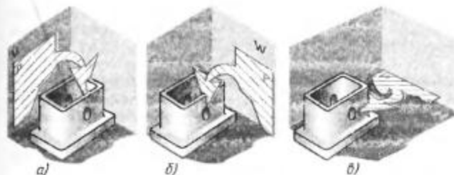
Рис. 181. Положение секущей плоскости при выполнении разреза
