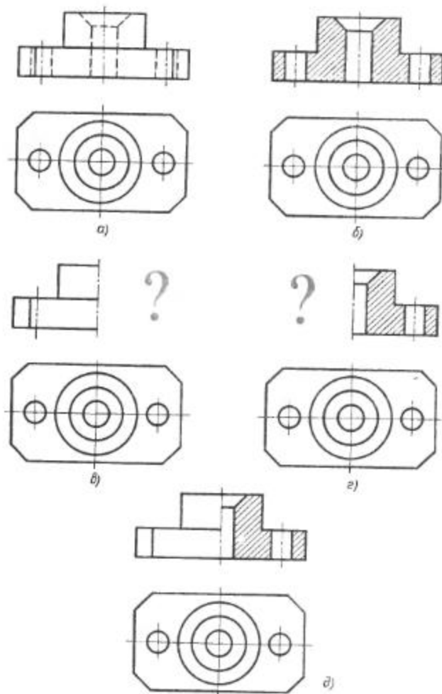
Рис. 192. Соединение половины вида и половины разреза
