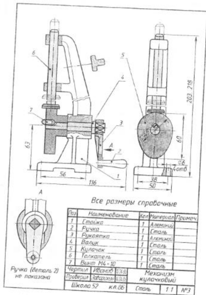
Рис. 232. Сборочный чертеж кулачкового механизма
