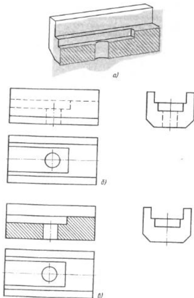
Рис. 178. Построение разреза
