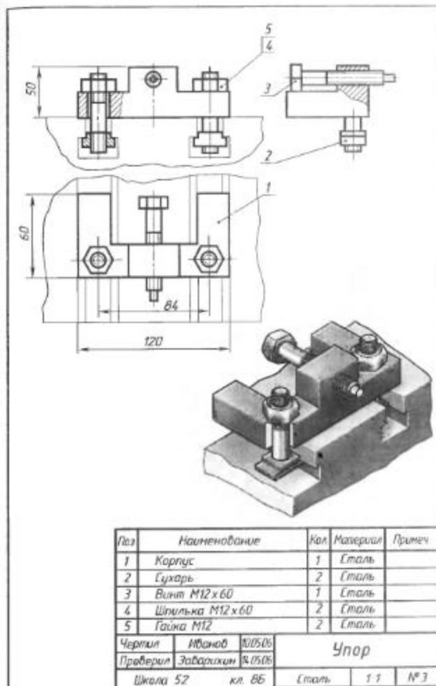
Рис. 250. Сборочный чертеж и наглядное изображение упора
