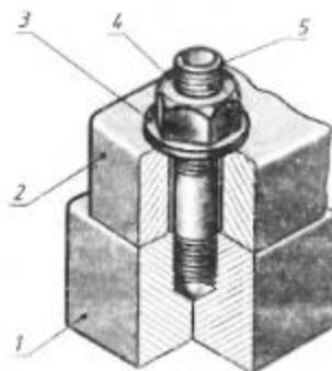
Рис. 218. Шпильчатое соединение
