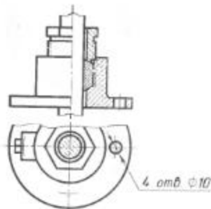
Рис. 242. Сальниковое устройство
