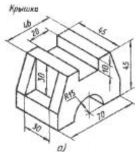
Рис. 158. Задание к графической работе № 10
