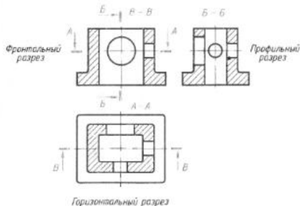
Рис. 182. Расположение и обозначение разрезов
