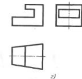
Рис. 111. Задания на проведение недостающих линий
