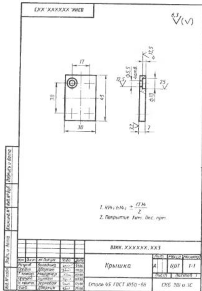
Рис. 4. Чертеж детали
