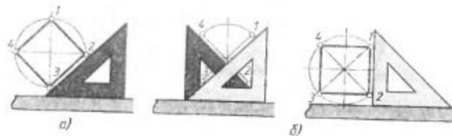
Рис. 124. Деление окружности на четыре равные части
