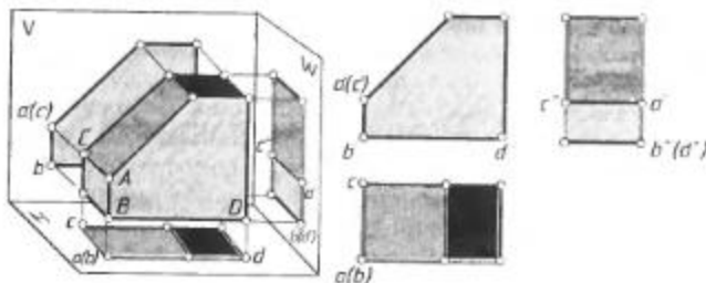
Рис. 86. Изображения предмета
