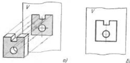
Рис. 43. Проецирование на одну плоскость проекций
