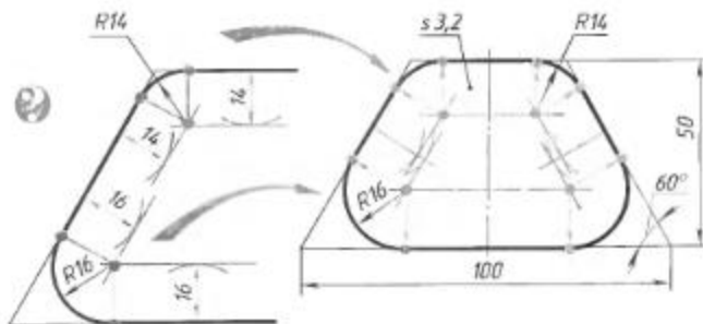
Рис. 134. Анализ контура изображения детали
