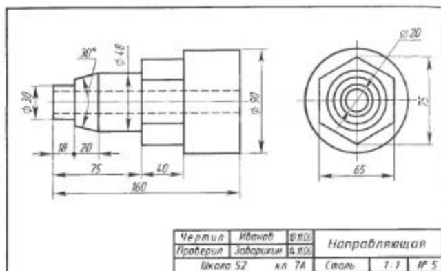
Рис. 143. Чертеж детали
