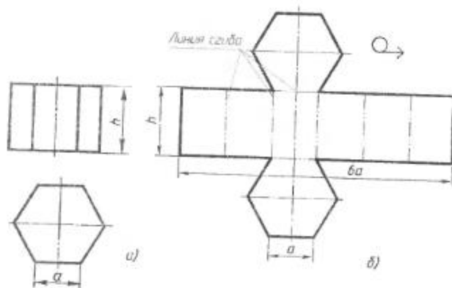
Рис. 139. Построение чертежа развертки поверхностей призмы: a — диаметр; b — развертка поверхностей
