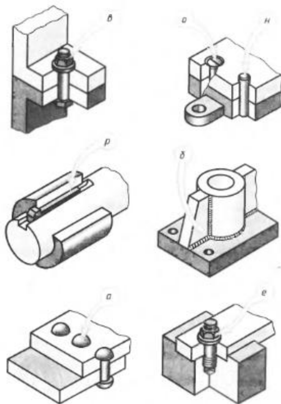
Рис. 209. Различные соединения деталей
