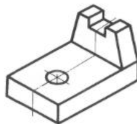
Рис. 9. Аксонометрический чертёж
