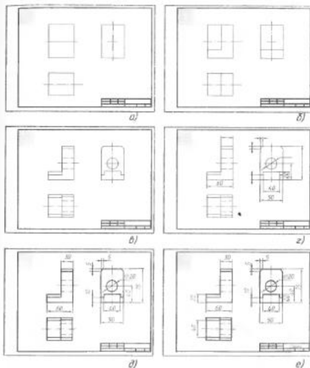
Рис. 154. Последовательность выполнения эскиза
