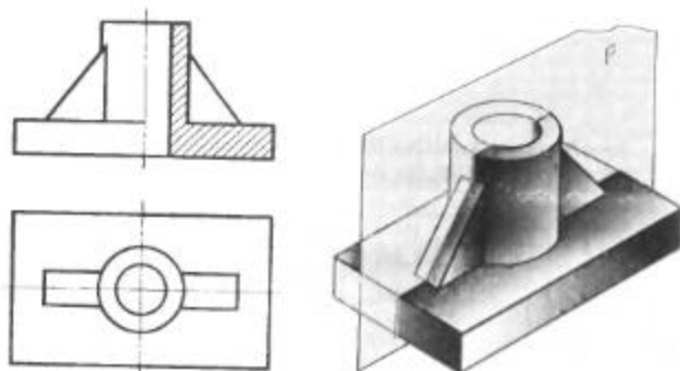
Рис. 196. Разрез вдоль тонкой стенки
