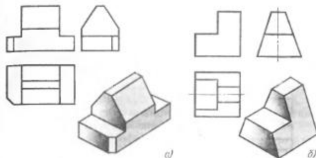
Рис. 88. Изображение элементов поверхности детали
