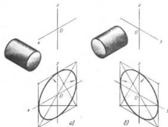
Рис. 67. Построение овалов:
