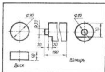
Рис. 158. Задание к графической работе № 10
