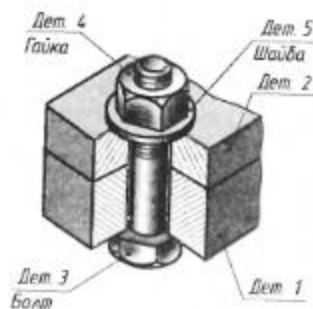
Рис. 216. Болтовое соединение
