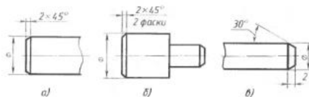
Рис. 118. Нанесение размеров фаски
