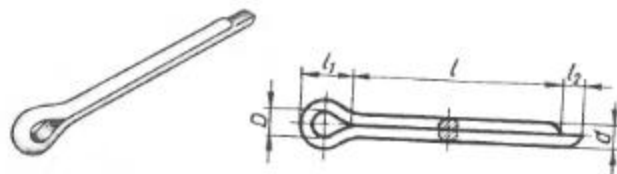
Рис. 252. Шпилька
