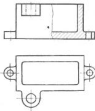
Рис. 191. Соединение частей вида и части разреза
