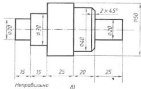
Рис. 117. Нанесение размеров
