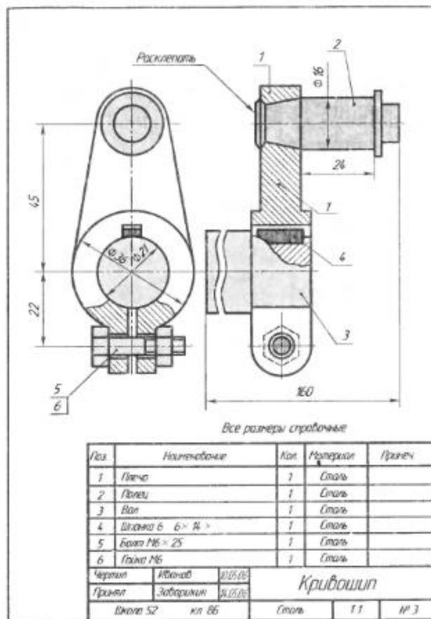
Рис. 254. Сборочный чертеж кривошипа
