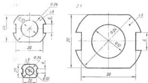
Рис. 35. Чертеж прокладки, выполненный в различных масштабах
