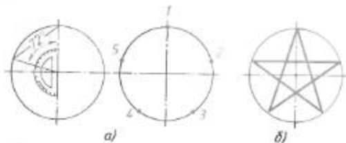
Рис. 129. Деление окружности на пять равных частей
