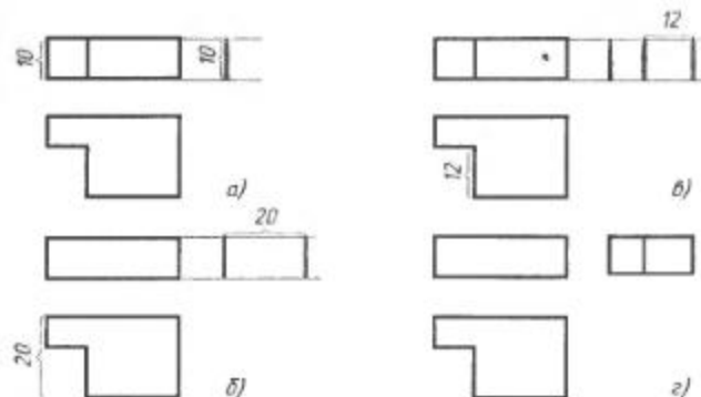
Рис. 109. Построение третьей проекции
