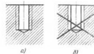
Рис. 221. Штриховка на изображении отверстия с резьбой: а — правильно; б — неправильно
