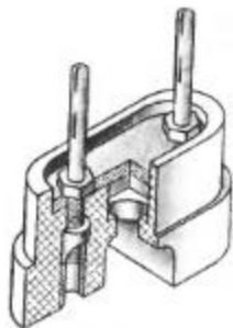
Рис. 241. Втулка
