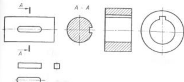
Рис. 224. Чертежи деталей шпоночного соединения
