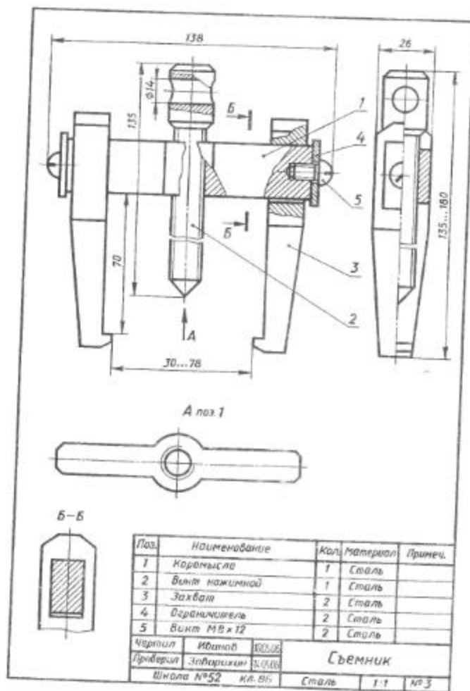
Рис. 245. Чертеж для чтения
