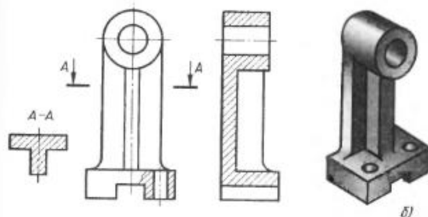
Рис. 165. Стойка
