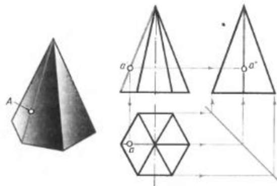
Рис. 91. Построение проекции точки, лежащей на ребре пирамиды
