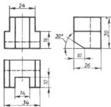
Рис. 103. Последовательность построения видов детали
