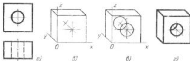
Рис. 64. Построение фронтальной диметрической проекции
