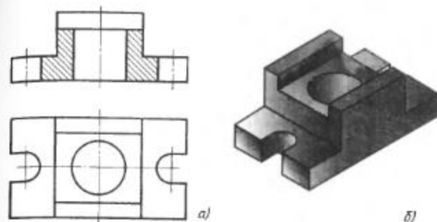
Рис. 164. Корпус
