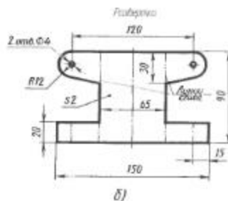
Рис. 8. Развертка и рисунок детали
