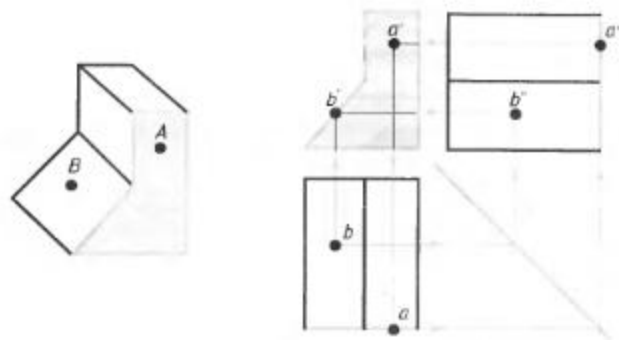
Рис. 93. Построение проекций точки, лежащей на поверхности предмета
