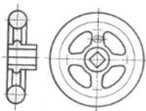
Рис. 197. Разрез детали со спицами
