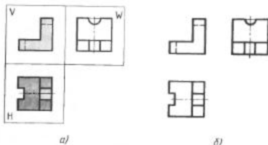
Рис. 50. Три проекции предмета
