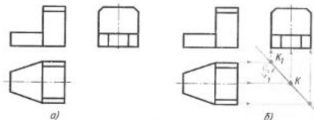
Рис. 92. Построение постоянной прямой
