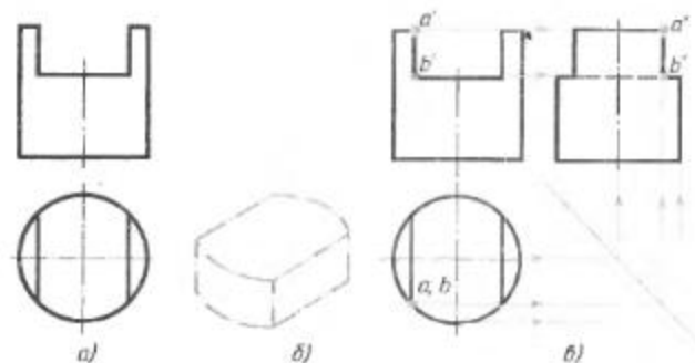
Рис. 106. Построение проекций детали, имеющей вырез
