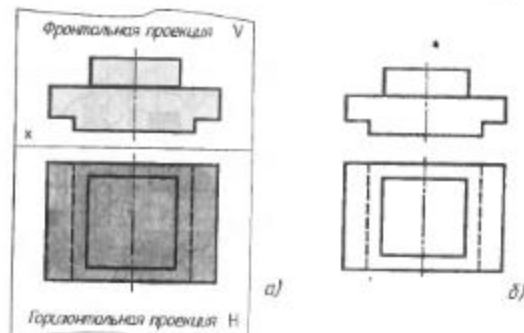
Рис. 47. Две проекции предмета
