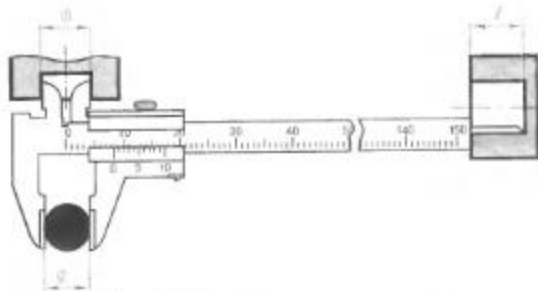
Рис. 153. Штангенциркуль
