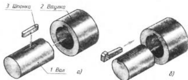
Рис. 222. Детали шпоночного соединения
