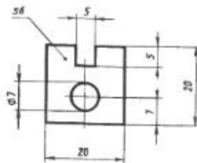
Рис. 44. Чертеж детали
