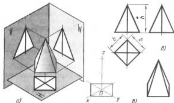
Рис. 79. Пирамиды:
