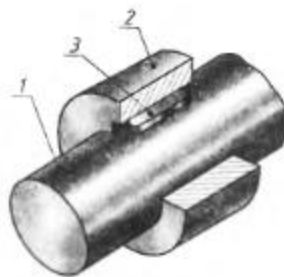
Рис. 223. Соединение шпонкой
