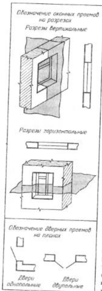
Рис. 262. Условные графические изображения оконных и дверных проемов
