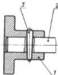
Рис. 229. Сборочный чертеж соединения
