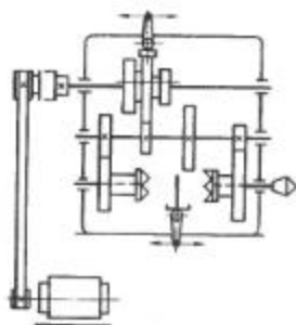
Рис. 7. Кинематическая схема
